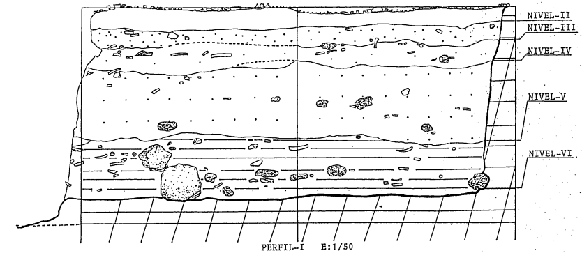
Fig. 6 a. Niveles edafológicos del Perfil I. Distintas densidades de material.
